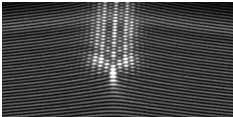
Figure 2 : Interférence d'un électron sur lui même
